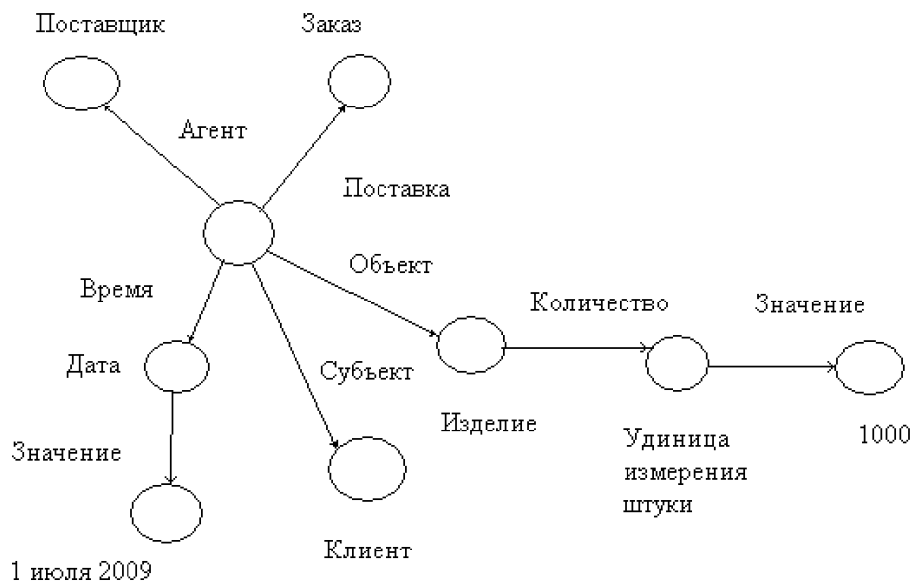
Рис. 1. Пример семантической сети
